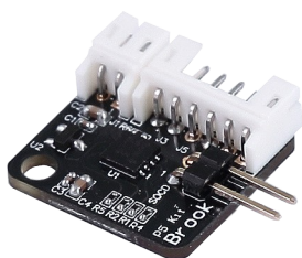
Kit de mise à niveau UFB (UFB-UP5) (L21 mm x L19,5mm x H6,6mm)
